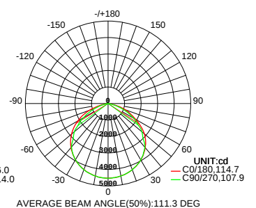
LF82R- 81W/13783lm
