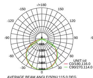
LF82R- 51W/8869lm
